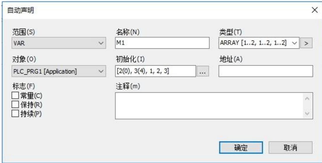
图 2-5-1 数组自动定义
