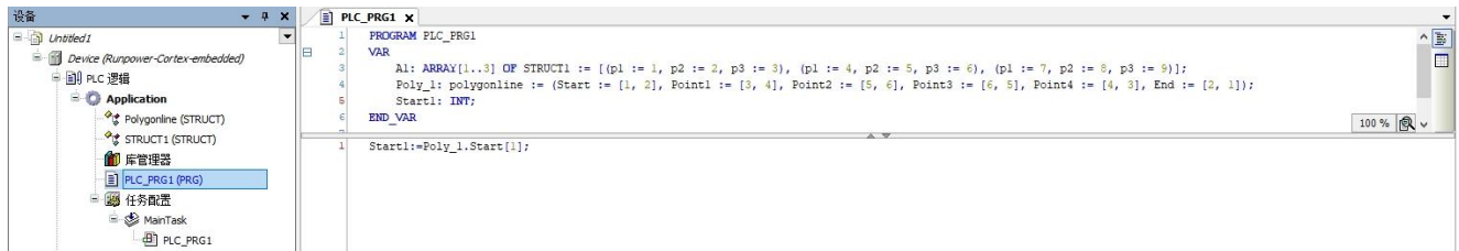
图 2-6-1 结构体定义举例
