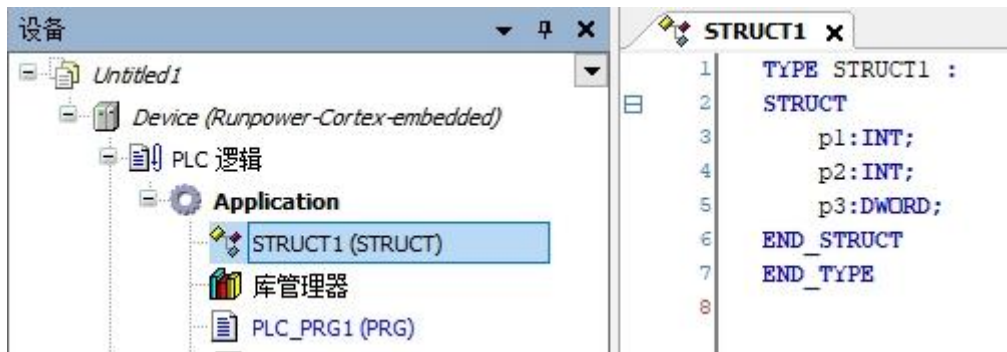
图 2-5-2 结构体定义
