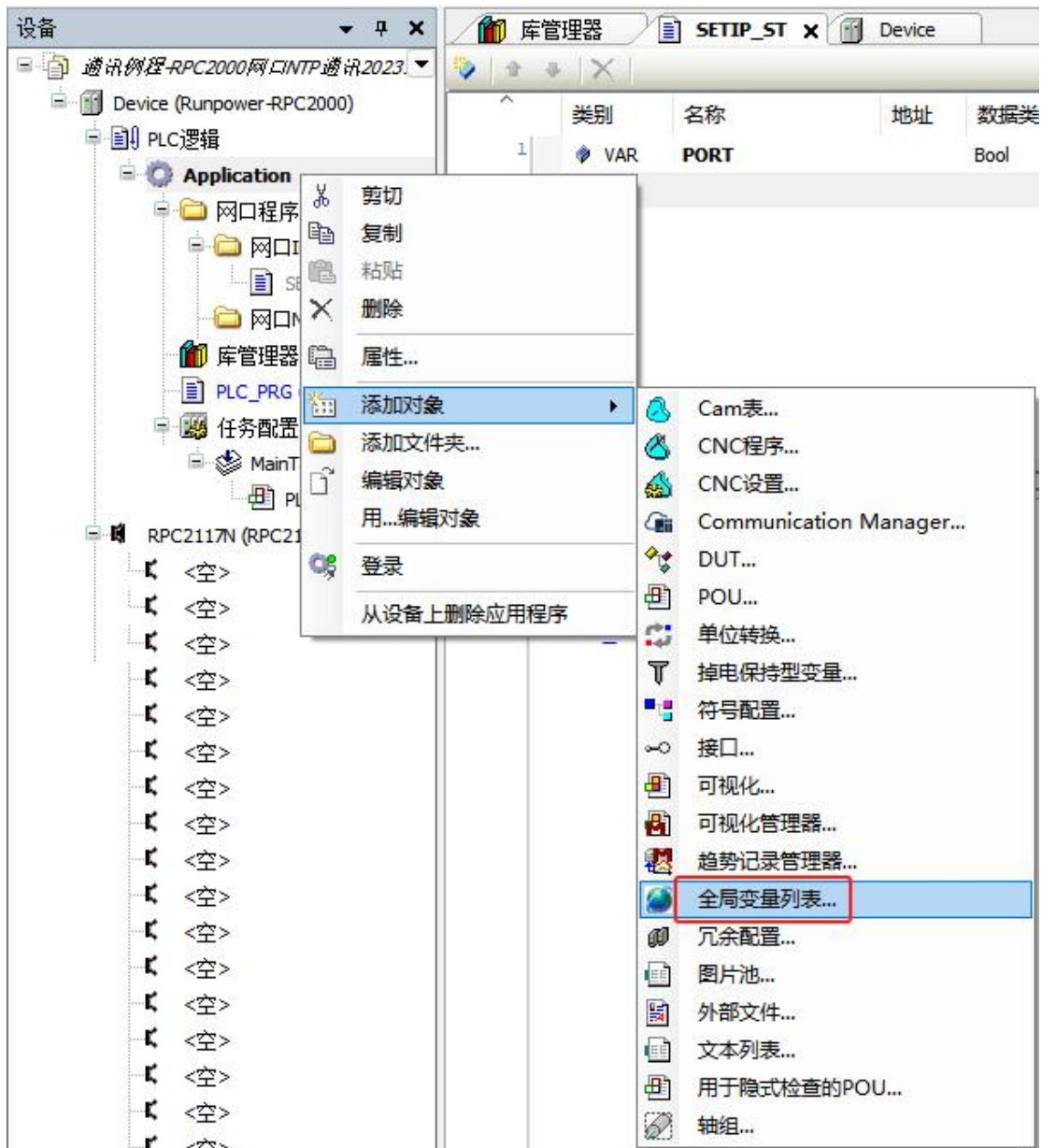
图 2-4-6 添加全局变量表
