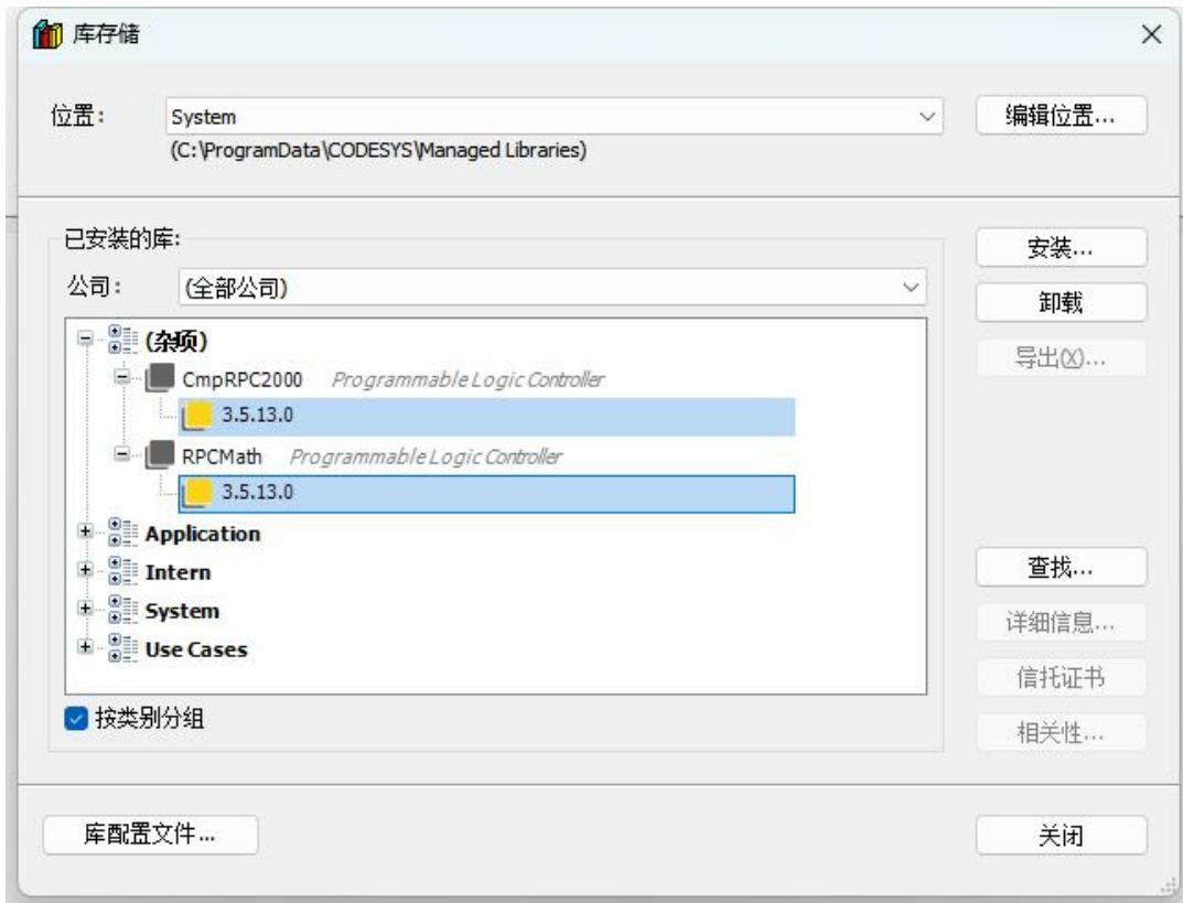
图 1-2-5 指令库安装步骤 5
